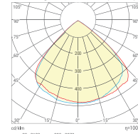
Косинусная КСС (Д90)
