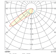
Асимметричная КСС (А50)
