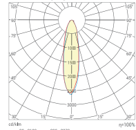
Концентрированная КСС
