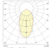
Глубокая КСС (Г60)
