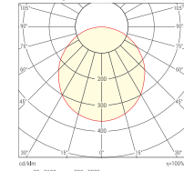
Косинусная КСС (Д120)
