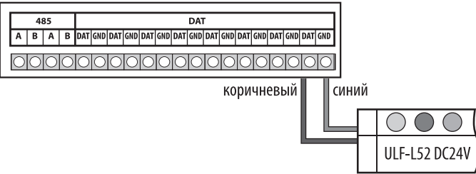
Рисунок 3. Схема подключения светильника к контроллеру.
