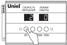
Рисунок 5. Пример изменения режима работы контроллера
