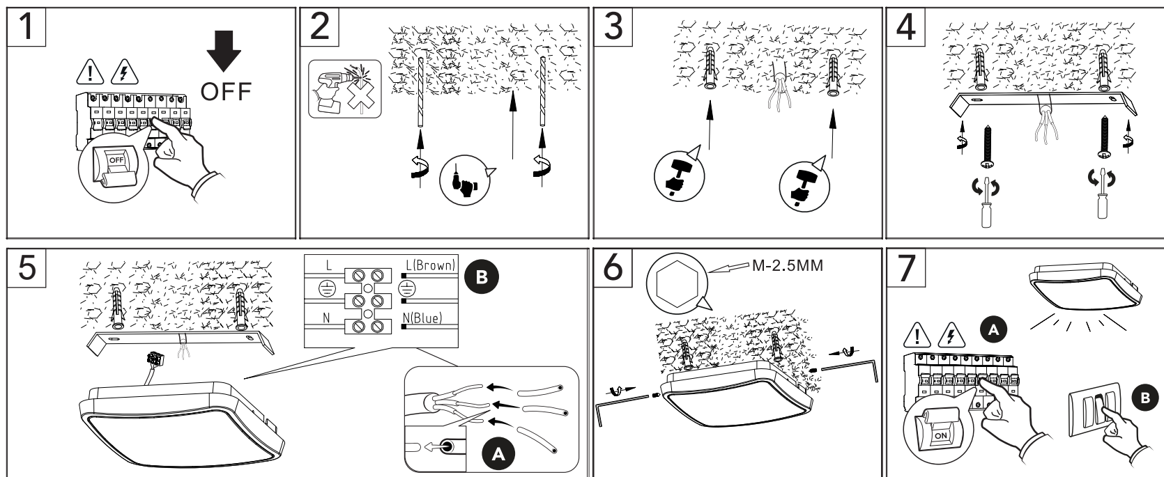
Схема монтажа
