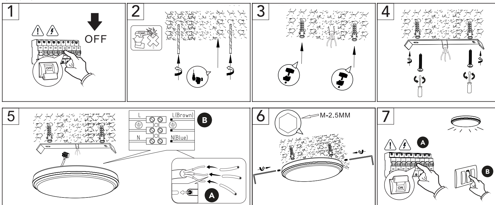
Схема монтажа
