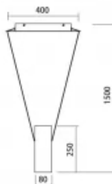
Габариты светильника
