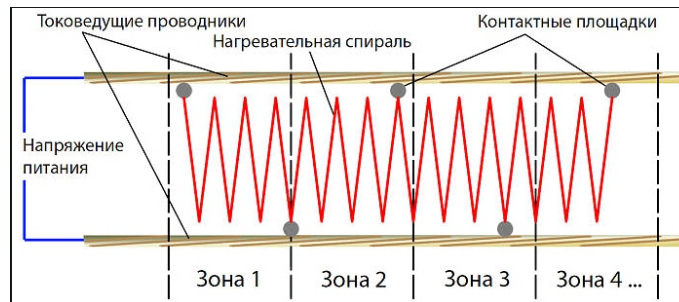
Рис. 16. Схема функционирования резистивного зонального кабеля..
