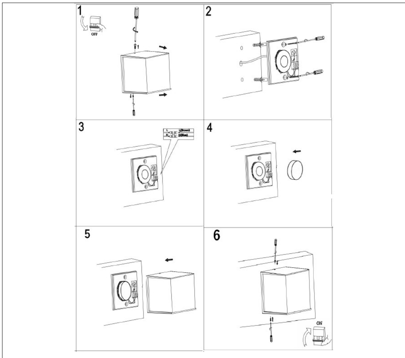
Рис. 1 Схема установки
