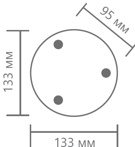
Рис. 1 Размеры основания светильника
