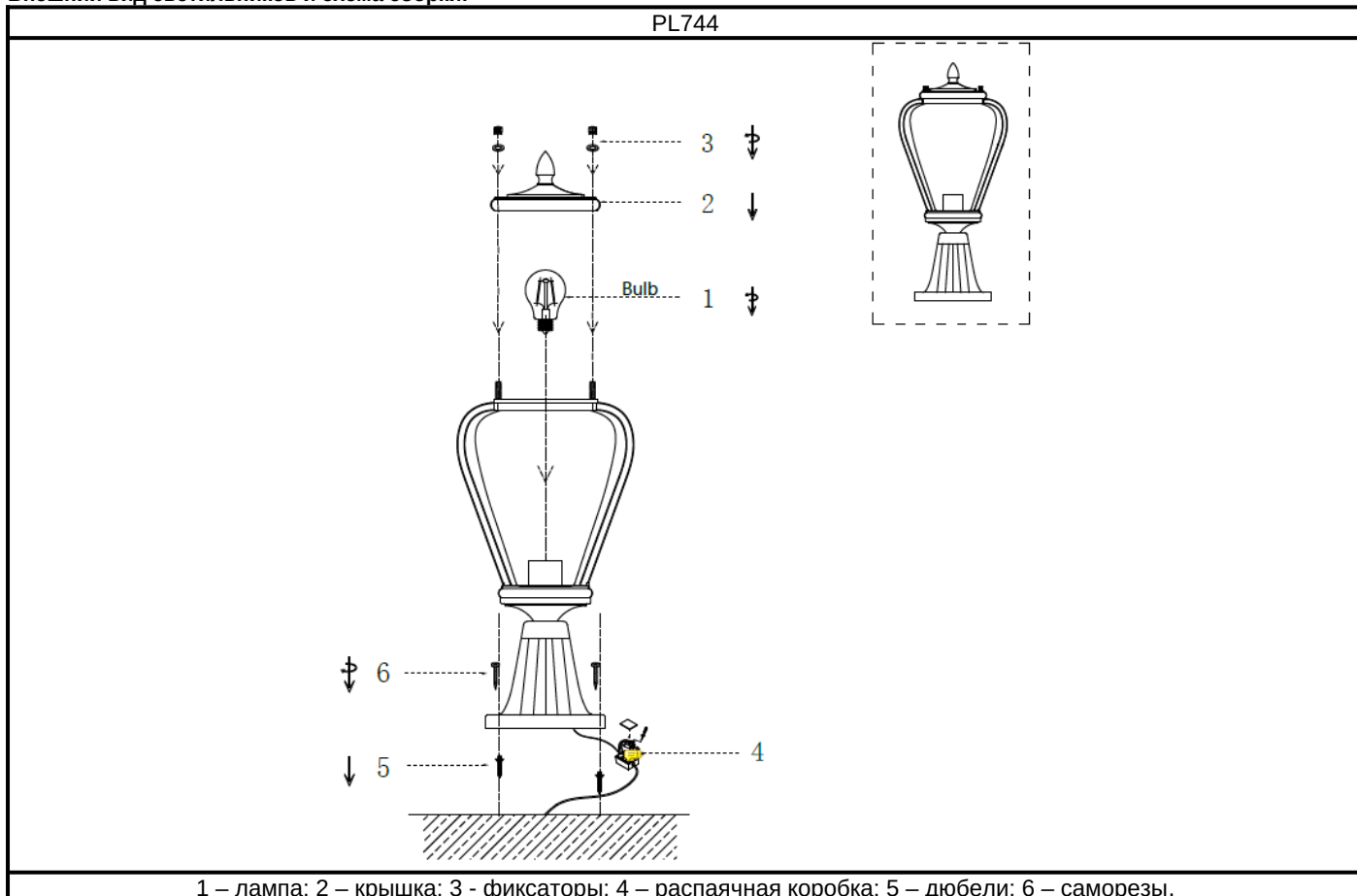
1 – лампа; 2 – крышка; 3 - фиксаторы; 4 – распаячная коробка; 5 – дюбели; 6 – саморезы.
