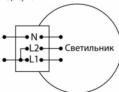
Рис. 2 Схема подключения
