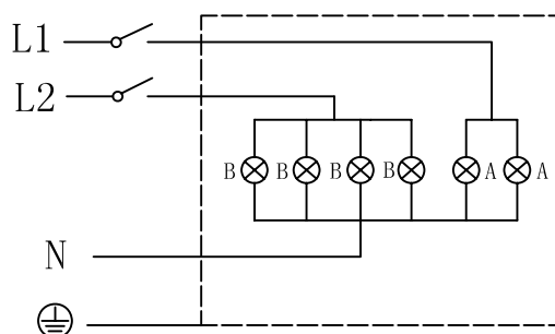
CIRCUIT SCHEMATIC принципиальная (электрическая) схема
