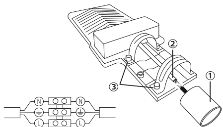
Рис. 1. Монтаж светильника
