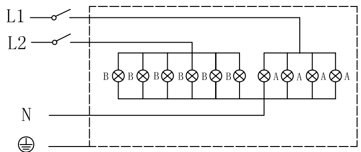
CIRCUIT SCHEMATIC принципиальная (электрическая) схема
